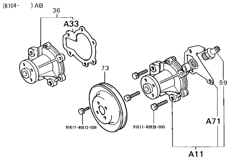
FIG.16-01 ウォータ ホップ
