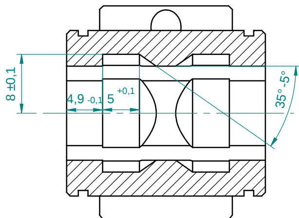
Schnitt A-A
